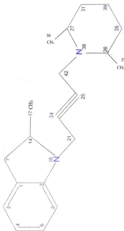
ANA4= (2R)-2-methyl-1,14-diazapentacyclo[3.3.1.0.0.0.0]nonane
